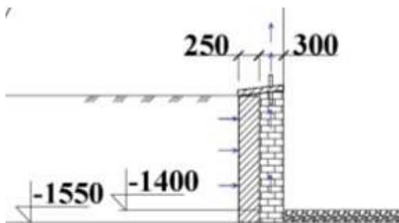
6-rasm. Majmuaning poydevorlari bo'lab qo'llanilgan “xataba” usulini sxematik ko'rinishi
