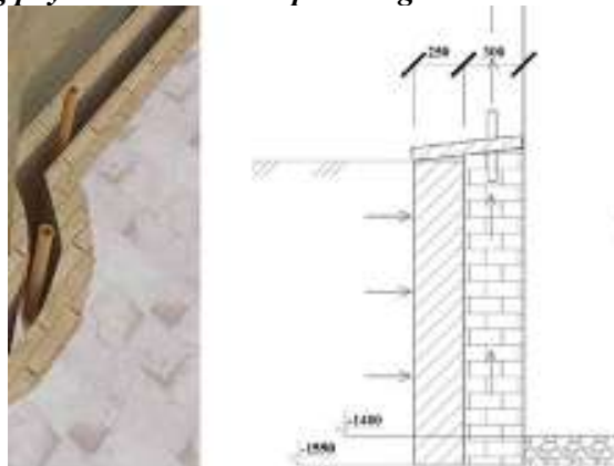
7-rasm. Majmuaning poydevorlari bo'lab qo'llanilgan “xataba” usulini sxematik ko'rinishi
