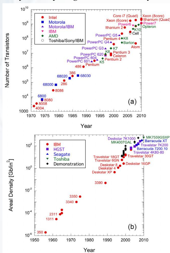
2-rasm. (a) Kremniy (Si) asosidagi protsessorlarda Mur qonuni. Yopiq doiralar, uchburchaklar, kvadratlar va romblar mos ravishda Intel, AMD, IBM va Motorola tomonidan ishlab chiqarilgan mikroprotsessorlarni ifodalaydi. (b) Qattiq disk (HDD)ning maydoniy
